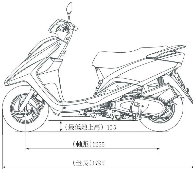
側面圖
