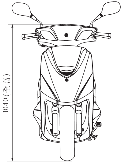
前面圖
