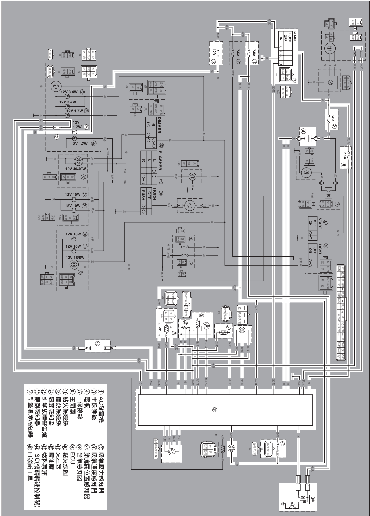
線路圖(32P2)
