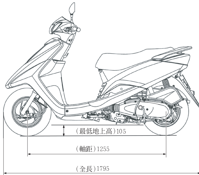
側面圖
