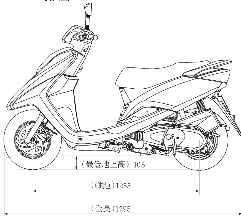
側面圖
